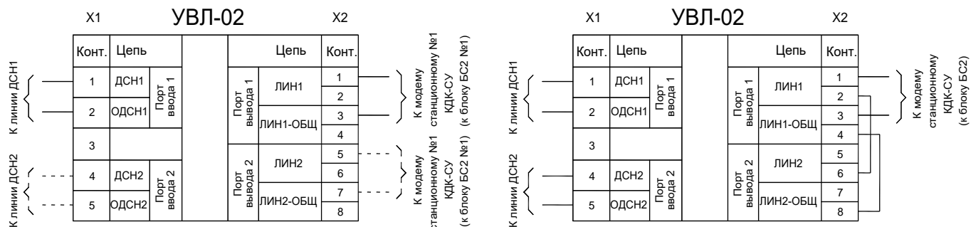
Рисунок 1 - Типовая схема подключения УВЛ-02 к одной или двум линиям связи (в том числе, к линиям ДСН) и одному или двум модемам стационарным КДК-СУ (блокам стационарным БС2)
